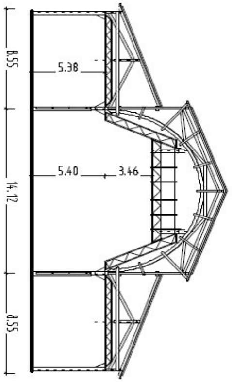
Schnitt quer
