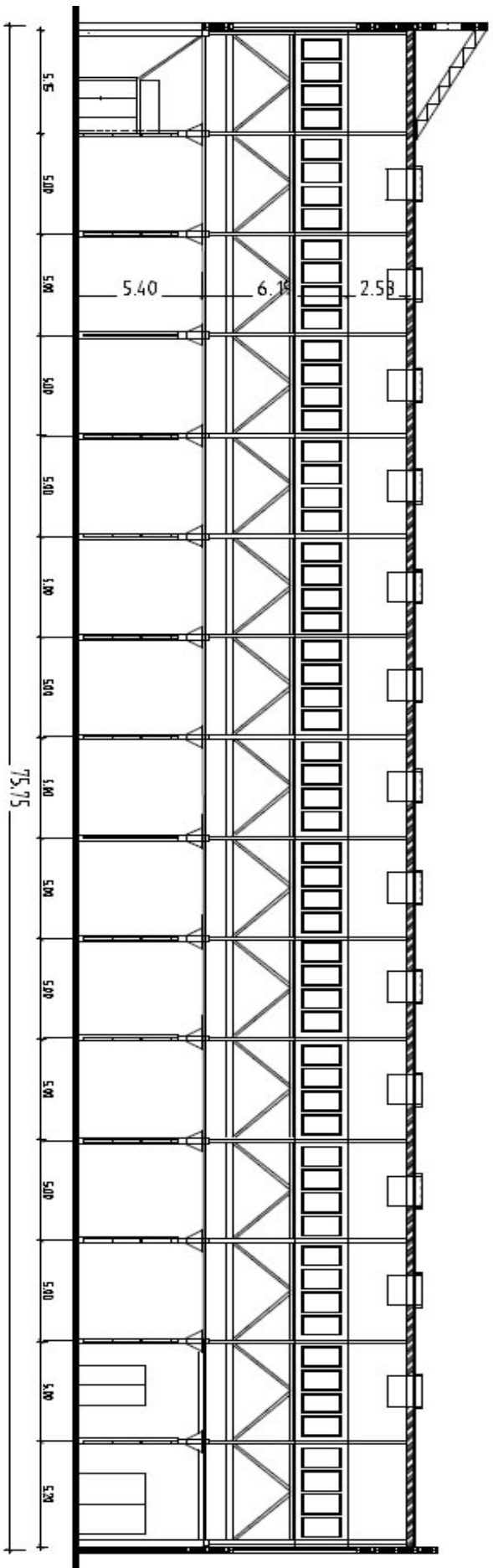
Schnitt längs
